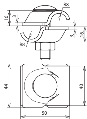
Maßbild MVK 16 16 FRM10X50 V2A
