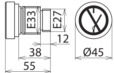
Maßbild SE E27 E33
