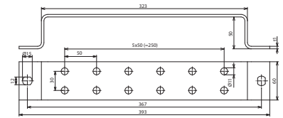
Maßbild ES 2X6 ASB11 STTZN
