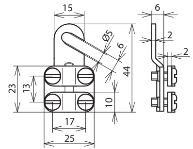
Maßbild EKSO 5.6 AQ6 16 CUGALZN
