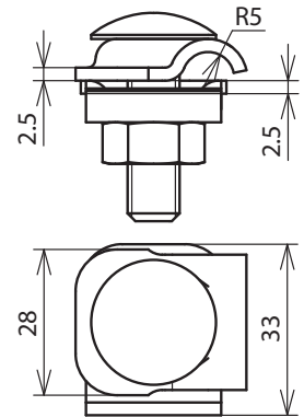
Maßbild MMVK 6.8 FRM10X35 STTZN
