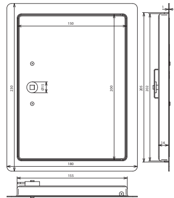
Maßbild RTUP 230X180 VKS STTZN
