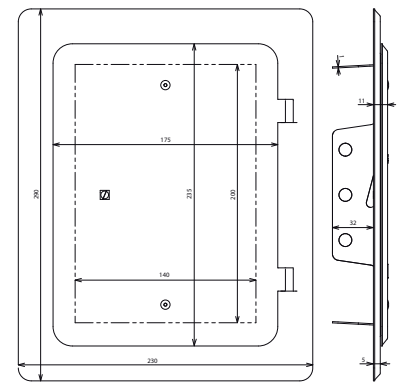
Maßbild RTUP 290X230 VKS V2A
