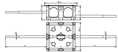
Maßbild TSK 140X140 V2A AF8 10 L200
