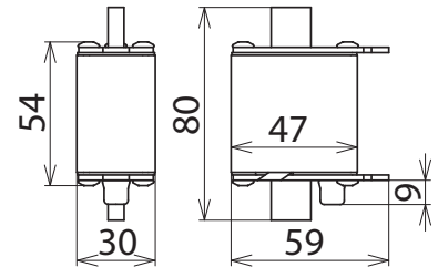
Maßbild V NH00 280
