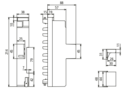
Maßbild DSH ZP B2 TNS 255
