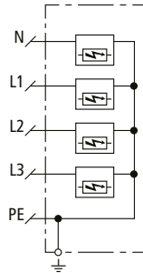
Prinzipschaltbild DSH ZP B2 TNS 255
