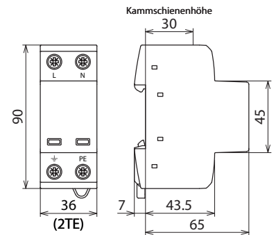
Maßbild DSH TN 255
