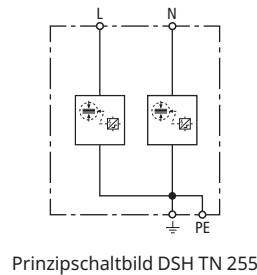
Prinzipialschaltbild DSH TN 255
