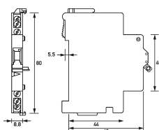
Maßzeichnung Gruppenansicht
