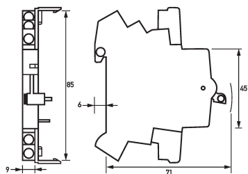
Maßzeichnung Gruppenansicht
