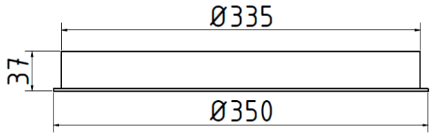
Maße Zentralbaldachin 350
