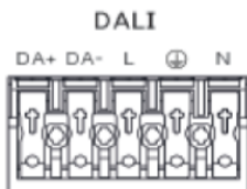
Abb.: 4 Anschlussschema: Dali oder schaltbar
