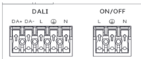
Abb.: 4 Anschlussschema: Dali oder schaltbar
