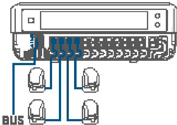
Beispielhafte Anschlusszeichnung
