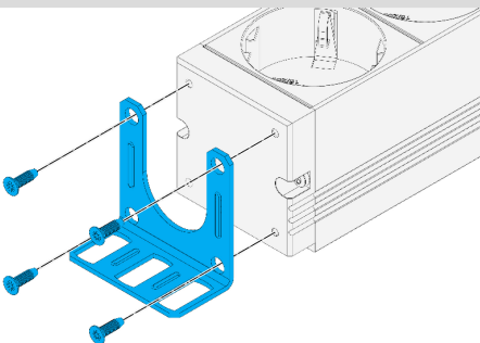
Haltewinkel montieren (4 Schrauben)
