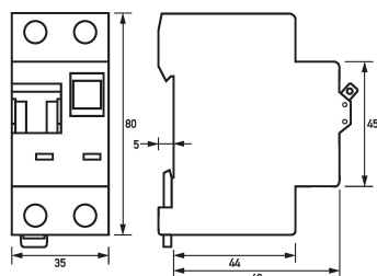
Maßzeichnung FI-/LS-Kombinationen DRCBO 3 B16/0,03/1N-A
